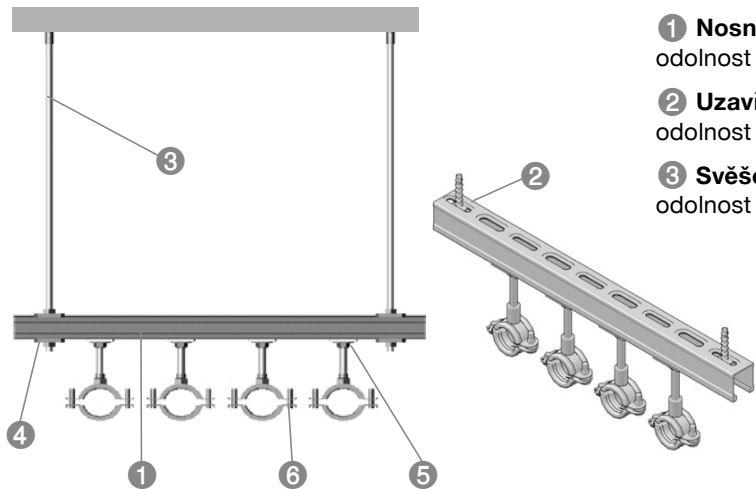
Závěsy typu: Hrazda s vodorovným nosníkem, nosník kotvený ke stropu
